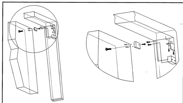
Схема за монтаж
